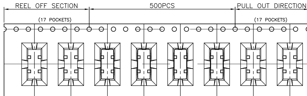
① 产品入载带示意图
