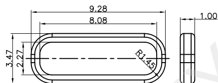
胶圈使用尺寸参考图
