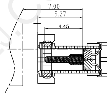
plug插入深度参考图
