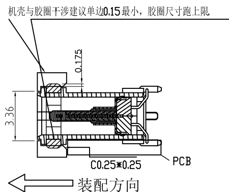
组装示意图
